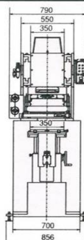
■XYθ付印刷テーブル寸法：350×250%
