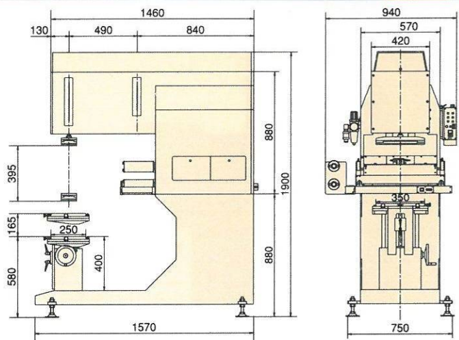
■XYθ付印刷テーブル寸法：350×250%
